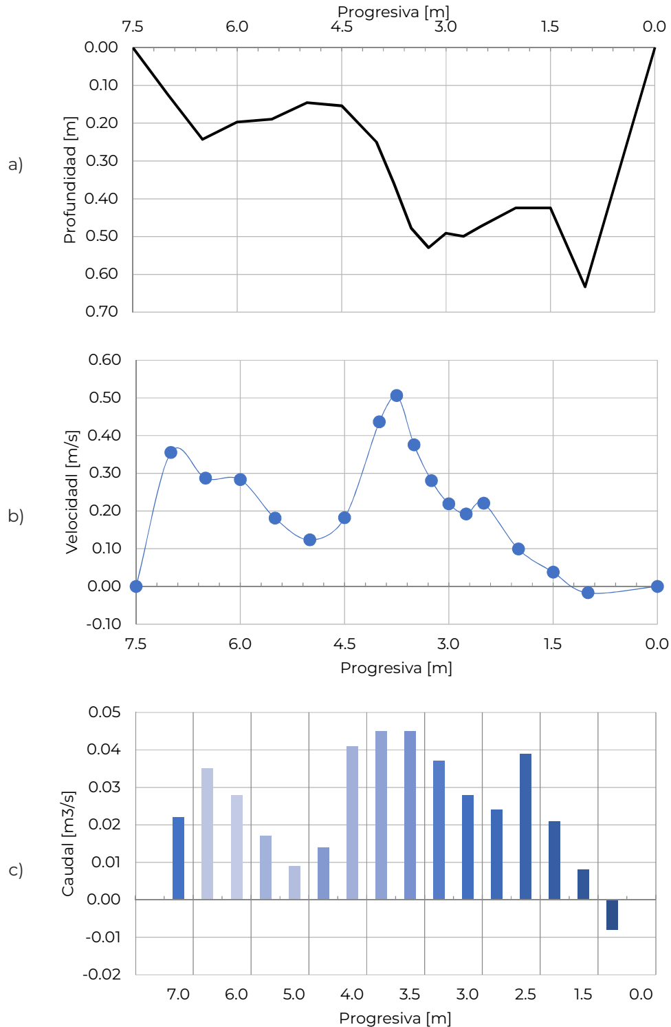
Figura 5. (a) Sección transversal del río Los Chorrillos en el sitio de medición, (b) perfil de velocidades medidos; (c) caudal aforado. La progresiva 0.00 corresponde con la margen derecha
