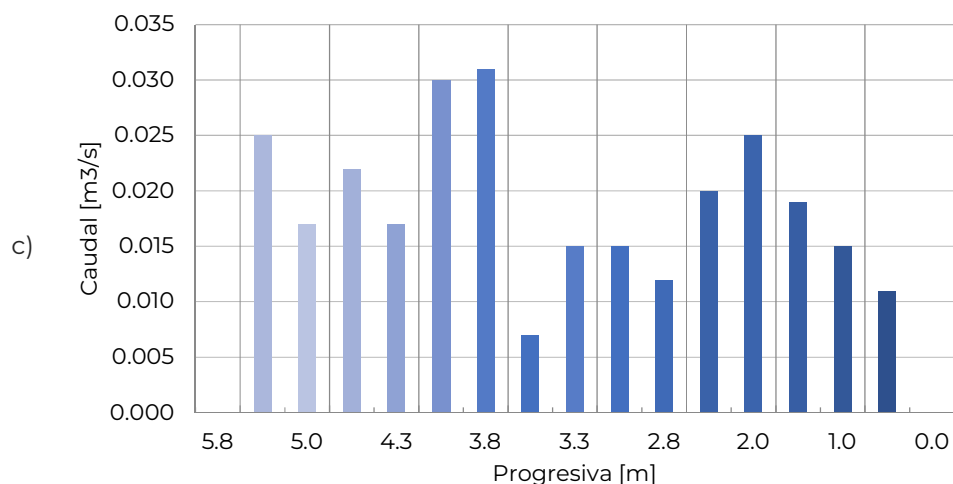
Figura 4. (a) Sección transversal del arroyo Las Mojaras en el sitio de medición (c) caudal aforado. La progresiva 0.00 corresponde con la margen izquierda
