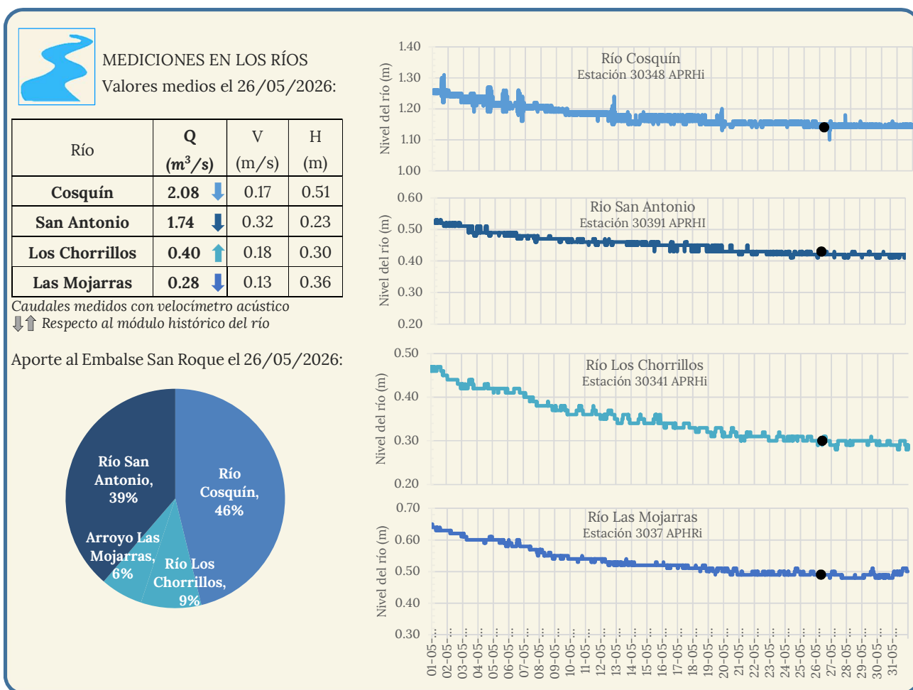
Figura 7. Resumen de las mediciones en los ríos el día 26/05/2026.
