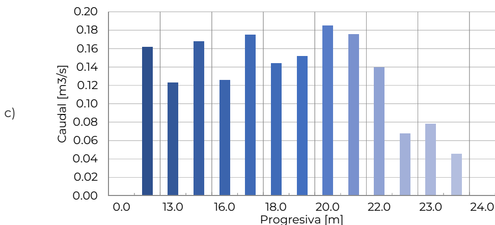
Figura 6. (a) Sección transversal del río San Antonio en el sitio de medición (b) perfil de velocidades medidos; (c) caudal aforado. La progresiva 0.00 corresponde con la margen izquierda
