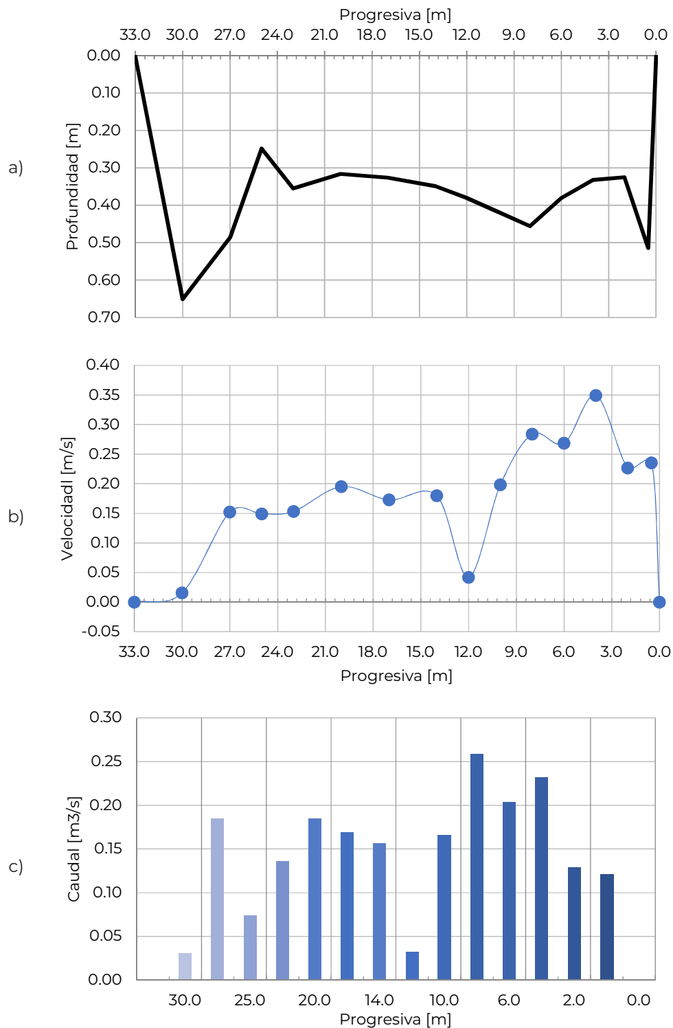
Figura 3. (a) Sección transversal del río Cosquín en el sitio de medición; (b) perfil de velocidades medidos; (c) caudal aforado. La progresiva 0.00 corresponde con la margen derecha
